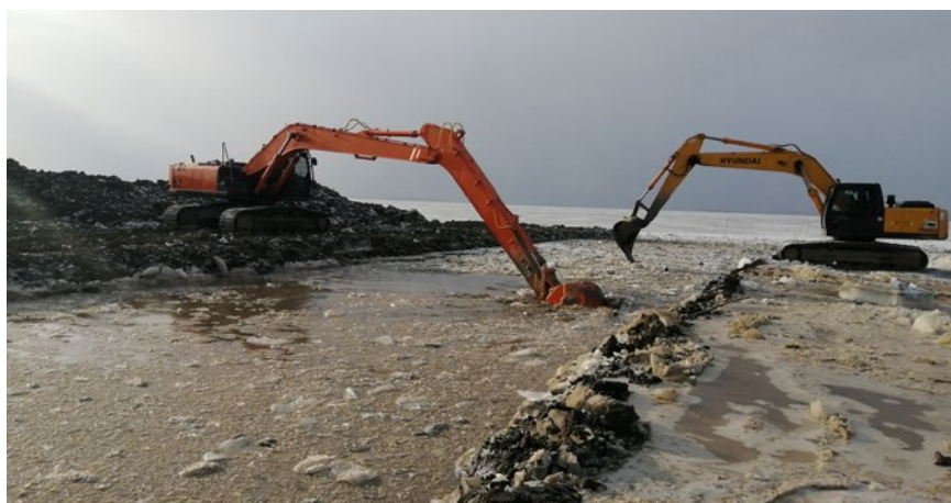
Магистральный газопровод «Сахалин–Хабаровск–Владивосток». Разработка подводной траншеи
